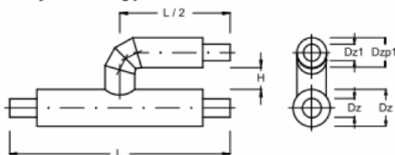
Trójnik równoległy
